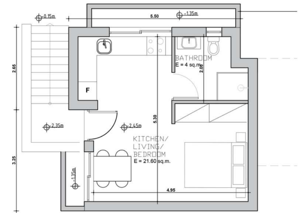
Plan : Semi-sous-sol - 21m 2
